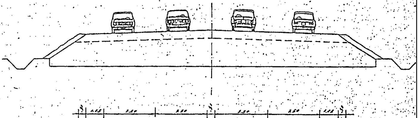
Il progetto della Modena-Sassuolo vista in sezione
